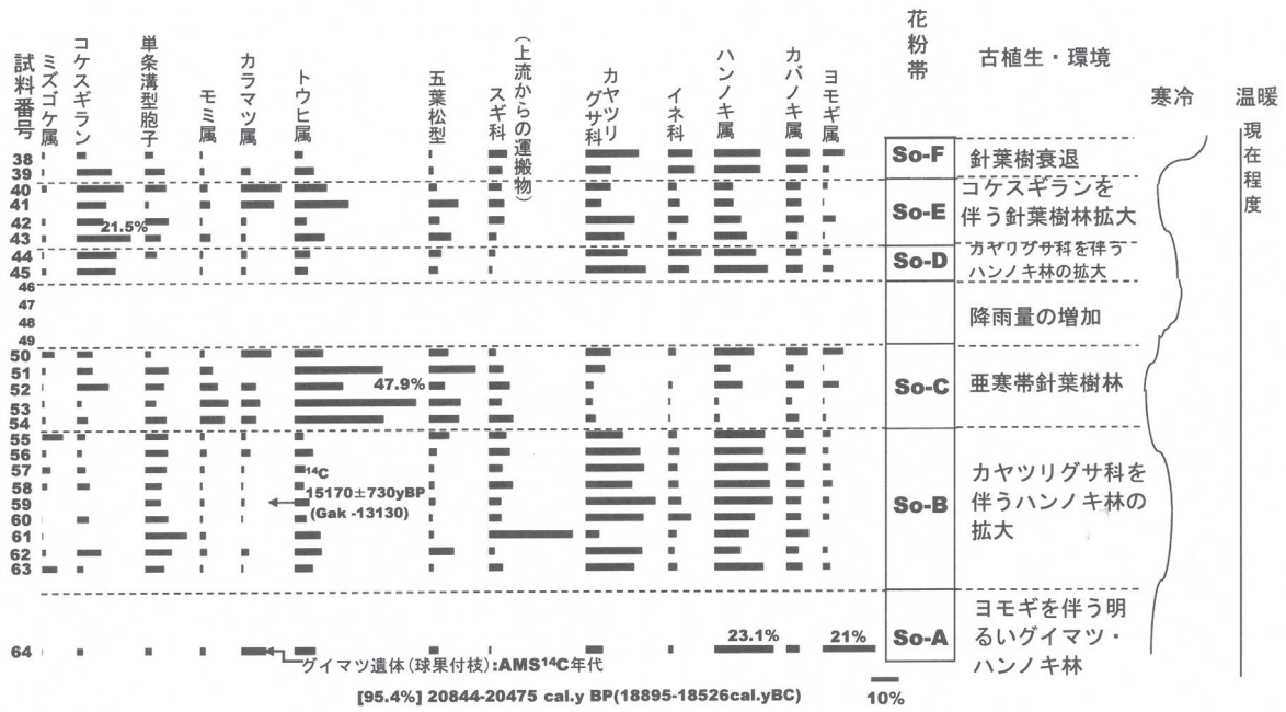
第 22 図 花粉・孢子組成図 (本文に示した理由により星野ほか, 2018 の図を改変)
