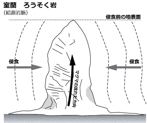
図 15 室蘭「ろうそく岩」の形成過程モデル
