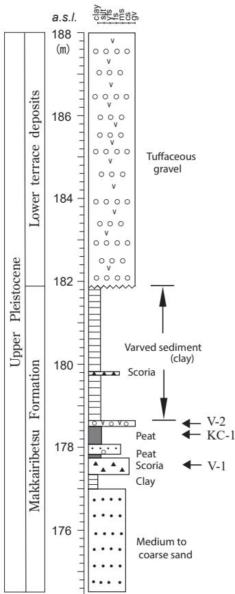
第3図 俱知安町市街南の露頭G-1の地質柱状図と試料採取点
