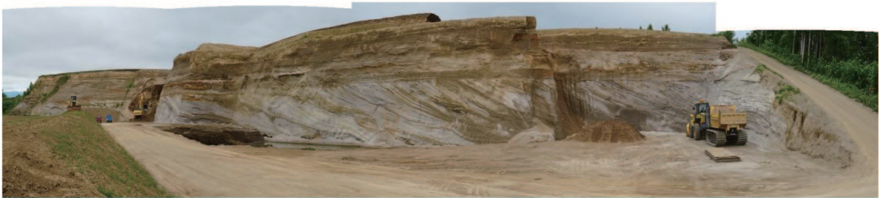
第6図 羊蹄山北麓の土取場 (露頭 G-4)
