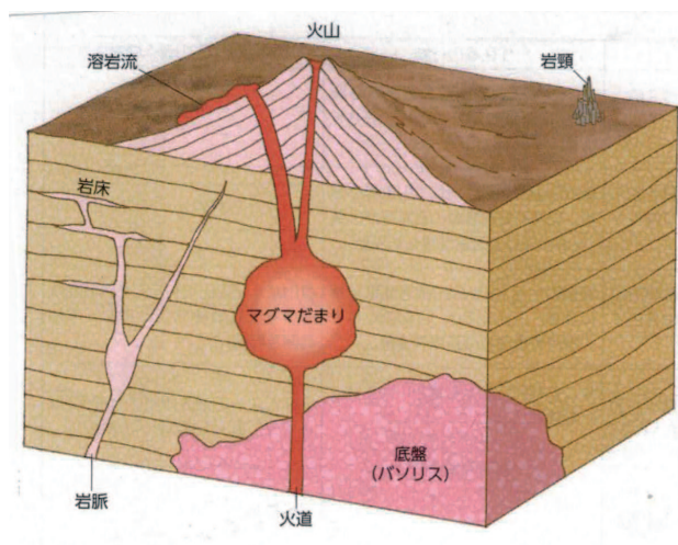
図1 岩脈と岩床：「ニューステージ地学図表」（浜島書店）（2021）より引用
