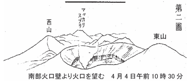
図8. 1874年火口と考えられる1901年溶岩ドーム形成前の火口(大井上, 1909)
