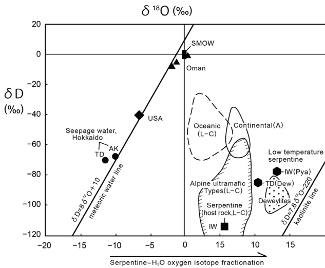
第9図 蛇紋岩関連の鉱物と水のδD-δ 18 O図(水落ほか, 2004). IW: 岩内岳 TD: 鷹泊 AK: 赤岩 Pya: パイロオーライト Dew: デュエライト L-C: リザルダイトークリソタイル A: アンチゴライト. 各エリアはO'Neil and Barnes (1971)をO'Hanley (1996)が修正. 北海道のデータは水落ほか(2004).
