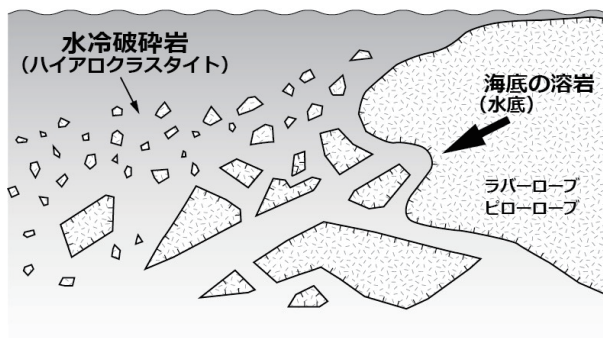
図5 水冷破碎岩(ハイアロクラスタイト)の形成
