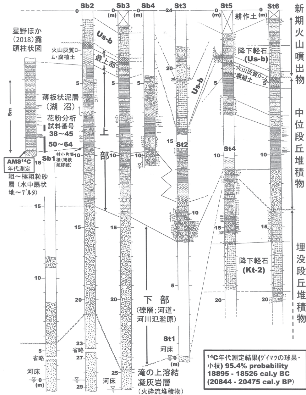
第 14 図 壮瞥橋～下立香橋南方面の中位段丘堆積物などの柱状対比図
