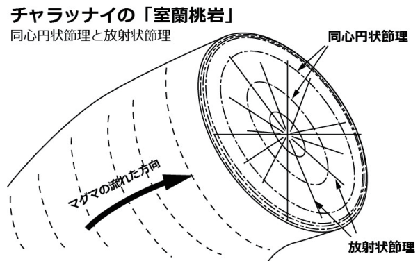
図 17 「室蘭桃岩」に見られる節理とその立体的イメージ
