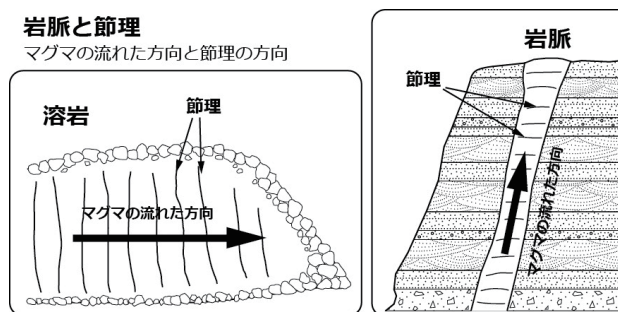
図2 岩脈と節理
