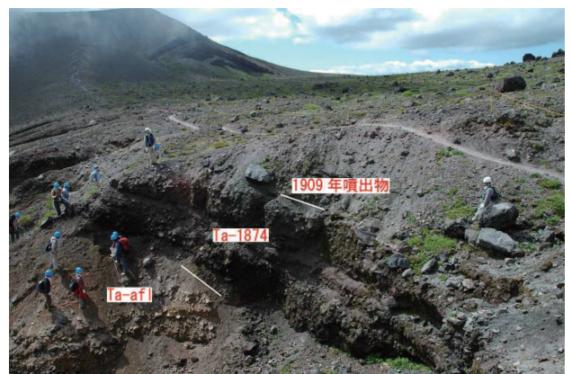
図9. 唐沢源頭の比較 [上] 1919年5月1日の樽前山山頂: 大井上(1919)の第8図 [下] 現在の唐沢源頭露頭: 中川(2011) 噴出物の境界を白線で示す。Ta-1874は1874年噴出物, Ta-afは1874年火砕流堆積物。左後方は西山, 背後に風不死岳。
