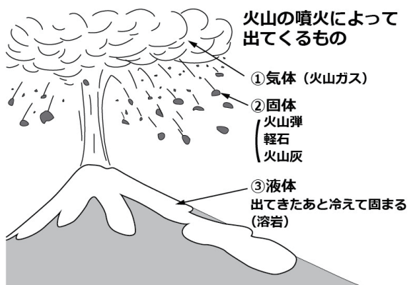
図6 火山から噴出するもの(火山噴出物)
